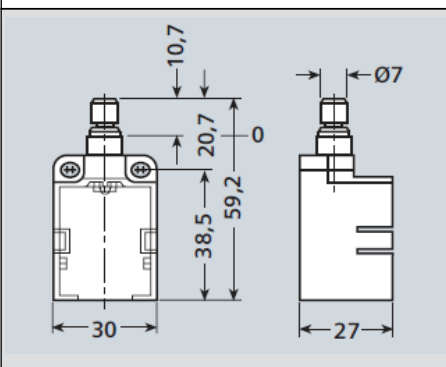
Caixa aberta 3SE5 250
