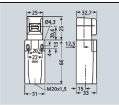
Caixa plástica largura de 31mm, 3SE5 23.-.QV40, 3SE5 23.-.RV40
