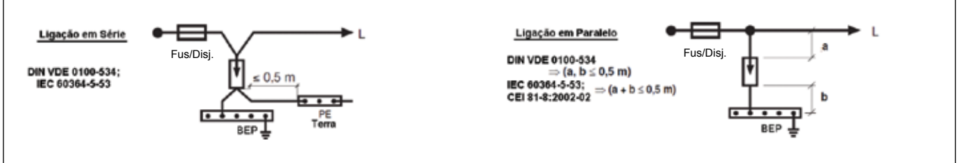
NBR 5410: 2004 - Figura 13 Esquemas de conexão dos DPS no ponto de entrada da alimentação de energia ou no quadro de distribuição da edificação
